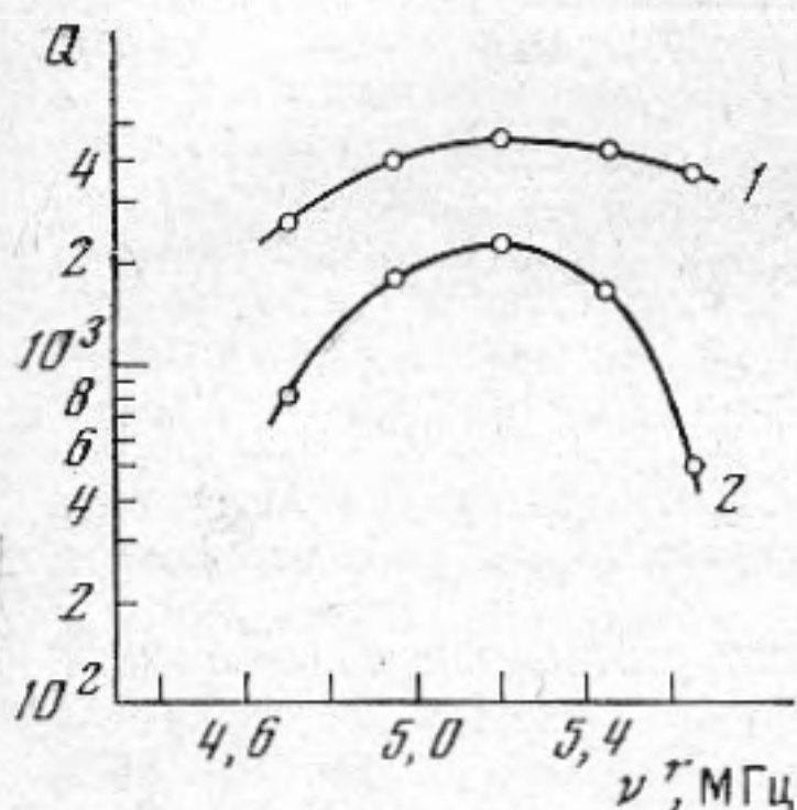
Фиг. 2. Зависимость добротности фильтра от частоты
