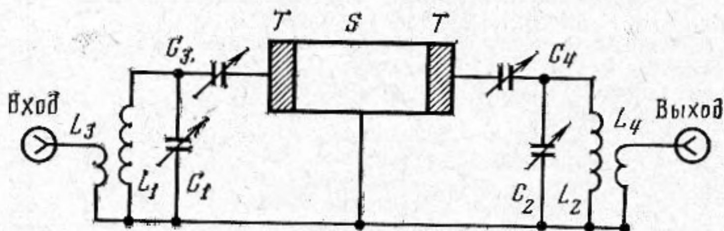
Фиг. 1. Схема акустического фильтра
