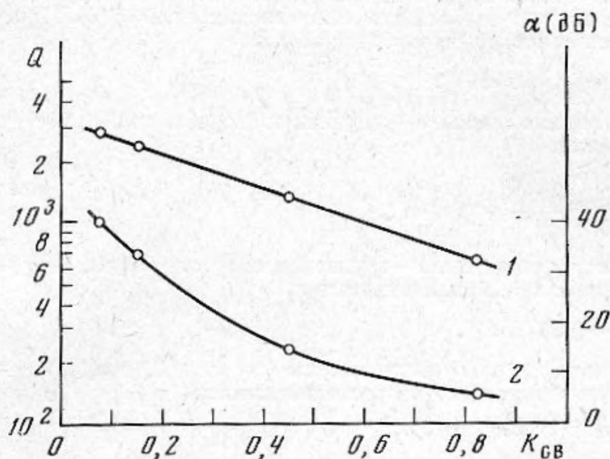
Фиг. 3. Зависимость добротности (кривая 1) и затухания (кривая 2) фильтра от коэффициента связи
