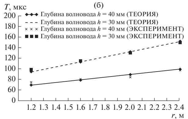
Рис. 7. Зависимость от длины трассы между источником и приемником (а) — времени вступления модовых импульсов и (б) — длительности принимаемого гидрофоном сигнала.
