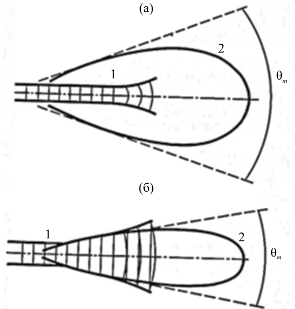
Рис. 1. Схема двух режимов работы параметрической антенны [6]: (а) — взаимодействие в ближней зоне первичного пучка; (б) — взаимодействие в его дальней зоне. Здесь 1 — первичный (высокочастотный) пучок, 2 — диаграмма направленности низкочастотного излучения. \theta_m — угловая ширина излучения.
