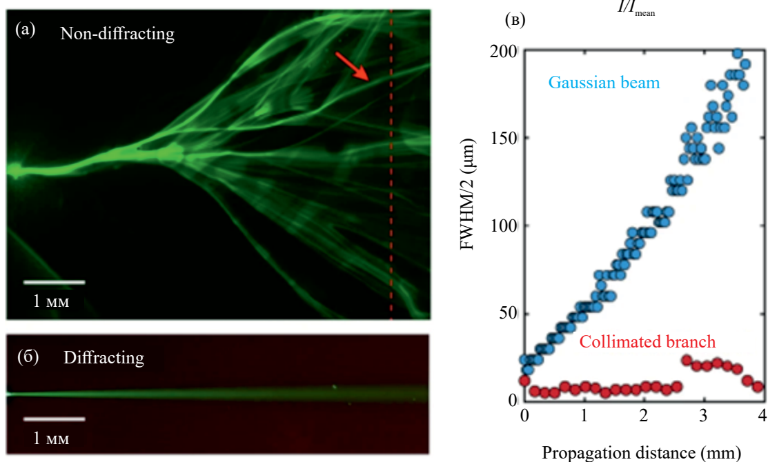
Рис. 8. Типичный вид ветвистого распространения в неоднородной среде [16]: (а) — иллюстрирует ограничение дифракции в каналах распространения сигнала, (б) — экспериментальное наблюдение дифракционного расширения гауссова пучка того же размера, что и в эксперименте (а), но в однородной среде, (в) — сравнение ширины пучка в канале, помеченном стрелкой на (а) с дифракционной шириной пучка в однородной среде на (б).
