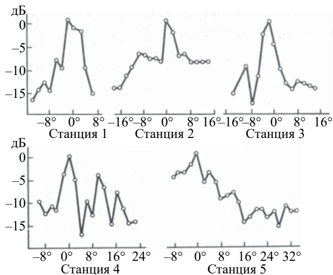
Рис. 4. Угловые характеристики акустических сигналов, прошедшие через вихрь по трассам, согласно станциям НИС АБК на рис. 3.
