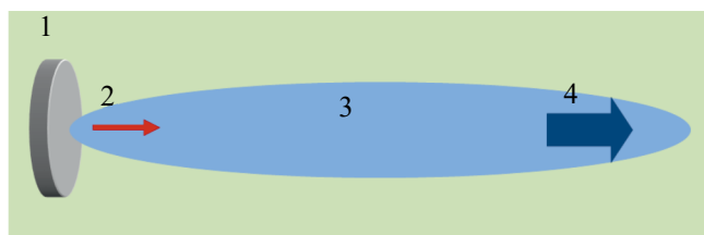
Рис. 1. Схема формирования сигнала параметрической антенной: 1 — излучатель высокочастотной накачки, 2 — излучение высокочастотной накачки, модулированной по интенсивности, 3 — область нелинейного акустического взаимодействия, 4 — низкочастотный сигнал параметрического излучения.
