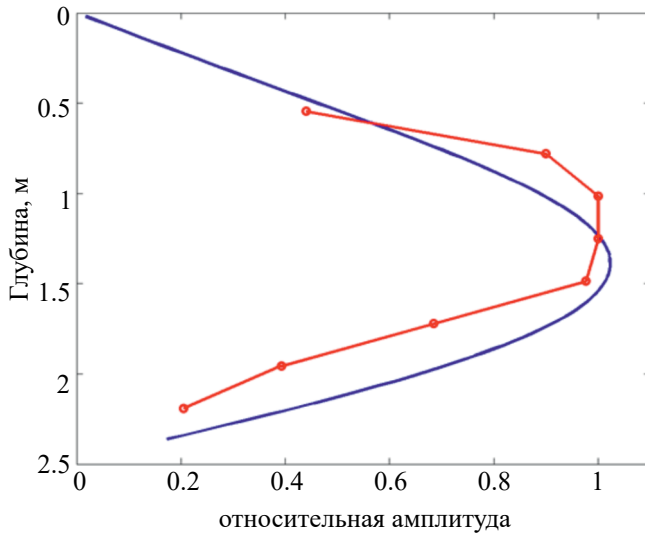
Рис. 5. Вертикальное распределение относительной амплитуды импульсов (красная) для частоты 15 кГц и 1-я мода собственной функции волновода (голубая) для экспериментального профиля звука и скорости звука в дне (продольной) 1600 м/с, плотность грунта 1700 кг/м 3 .
